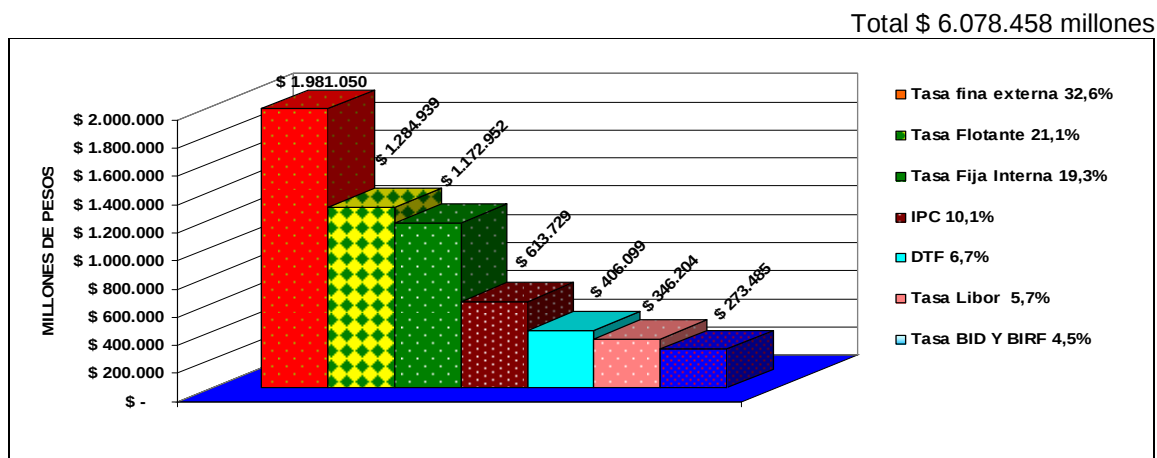
Gráfica 3 Distribución porcentual de la deuda a 30 de septiembre de 2010 Clasificada por tasas de interés
